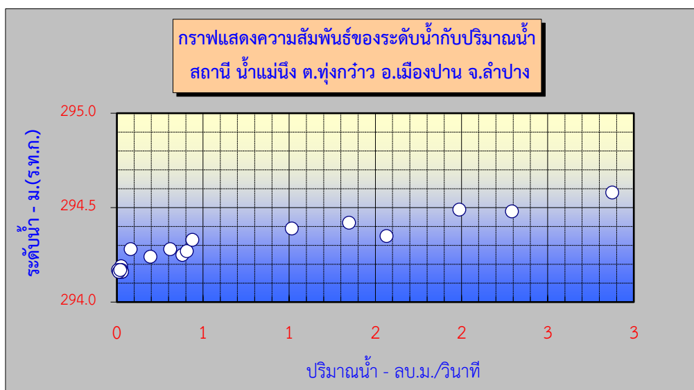
รูปที่ 13 กราฟแสดงความสัมพันธ์ของระดับน้ำกับปริมาณน้ำสถานี น้ำแม่เนื่อง บ้านป่าเวียง อ.เมืองปาน จ.ลำปาง
